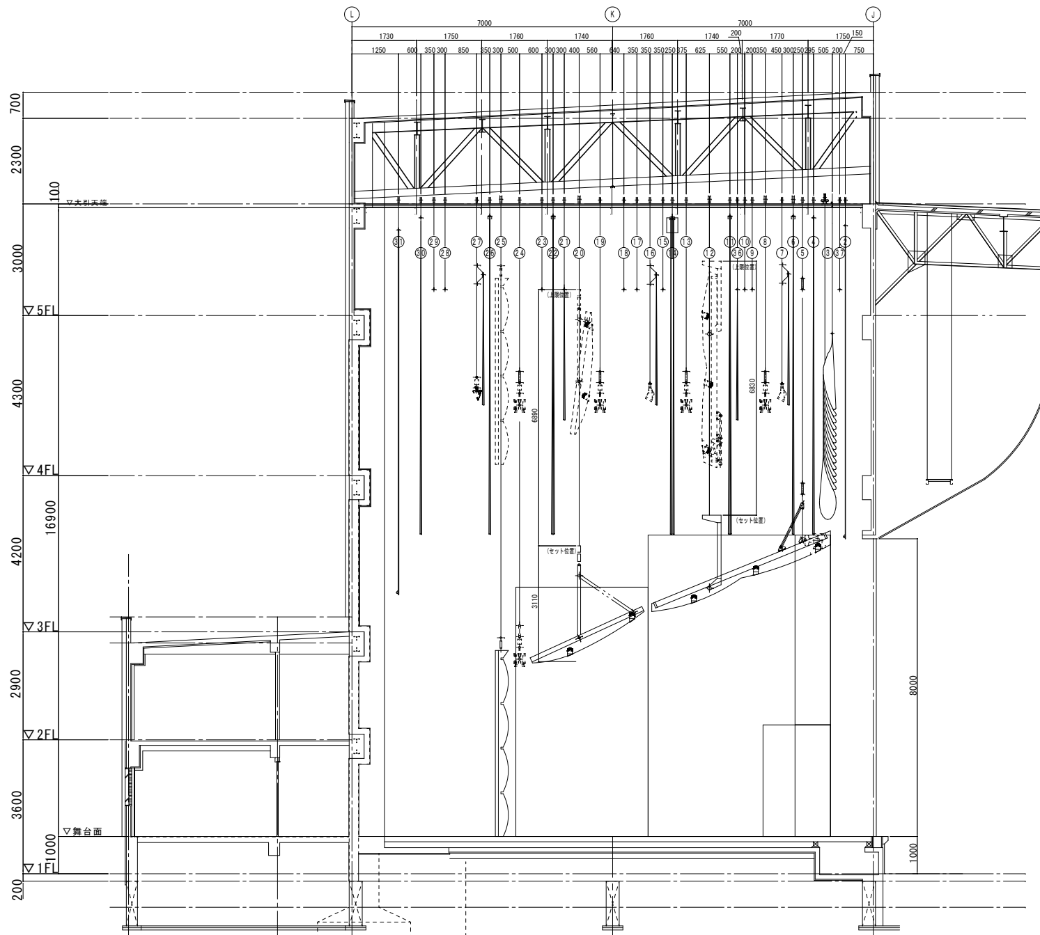
北見市民会館大ホール舞台断面図
