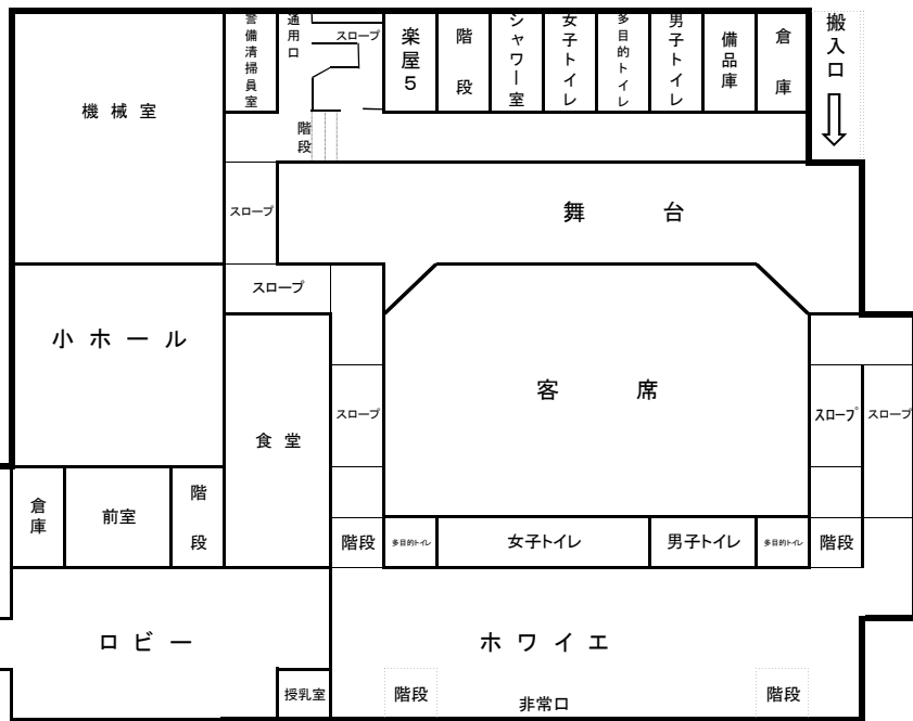
( 1 階 平 面 図 )
